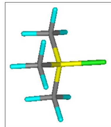
produkt
