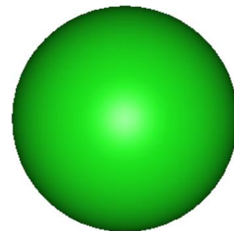
klorid ion
