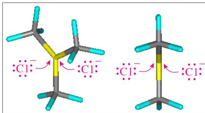
karbokation
