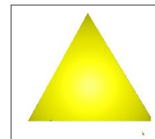
otkriveni dio atoma ugljika u SN1 reakciji
